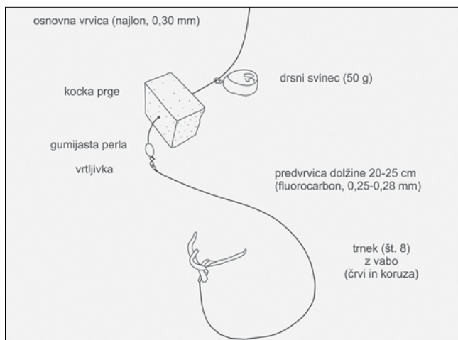
Sl. 1. Sistem talnega ribolova s kocko prge namesto krmilnika (risba: B. Kramberger).
