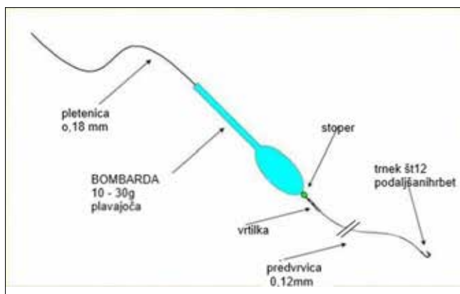
Sistem z bombardo (namesto trnka lahko uporabite silikonsko ribico ali prejico).
